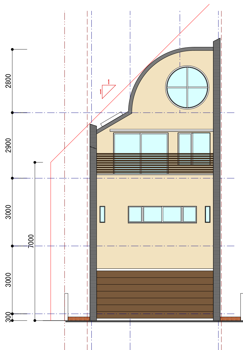
北側立面図
